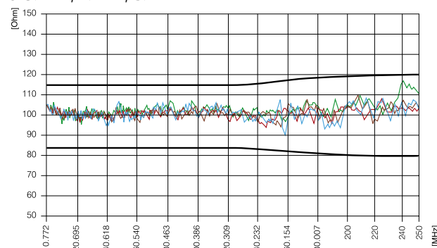
Typowa charakterystyka impedancji falowej kabli kat. 6 U/FTP, F/FTP, S/FTP
